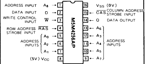
Outline 16P4H(DIP)
