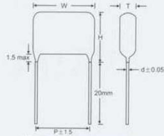
外形圖 Outline Drawing
