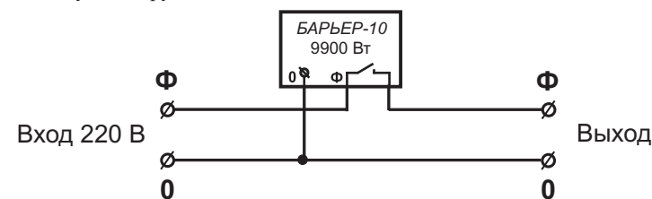
Рис.1 Схема подключения прибора.
