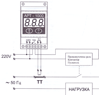
Рис.1 Вариант подключения прибора.
